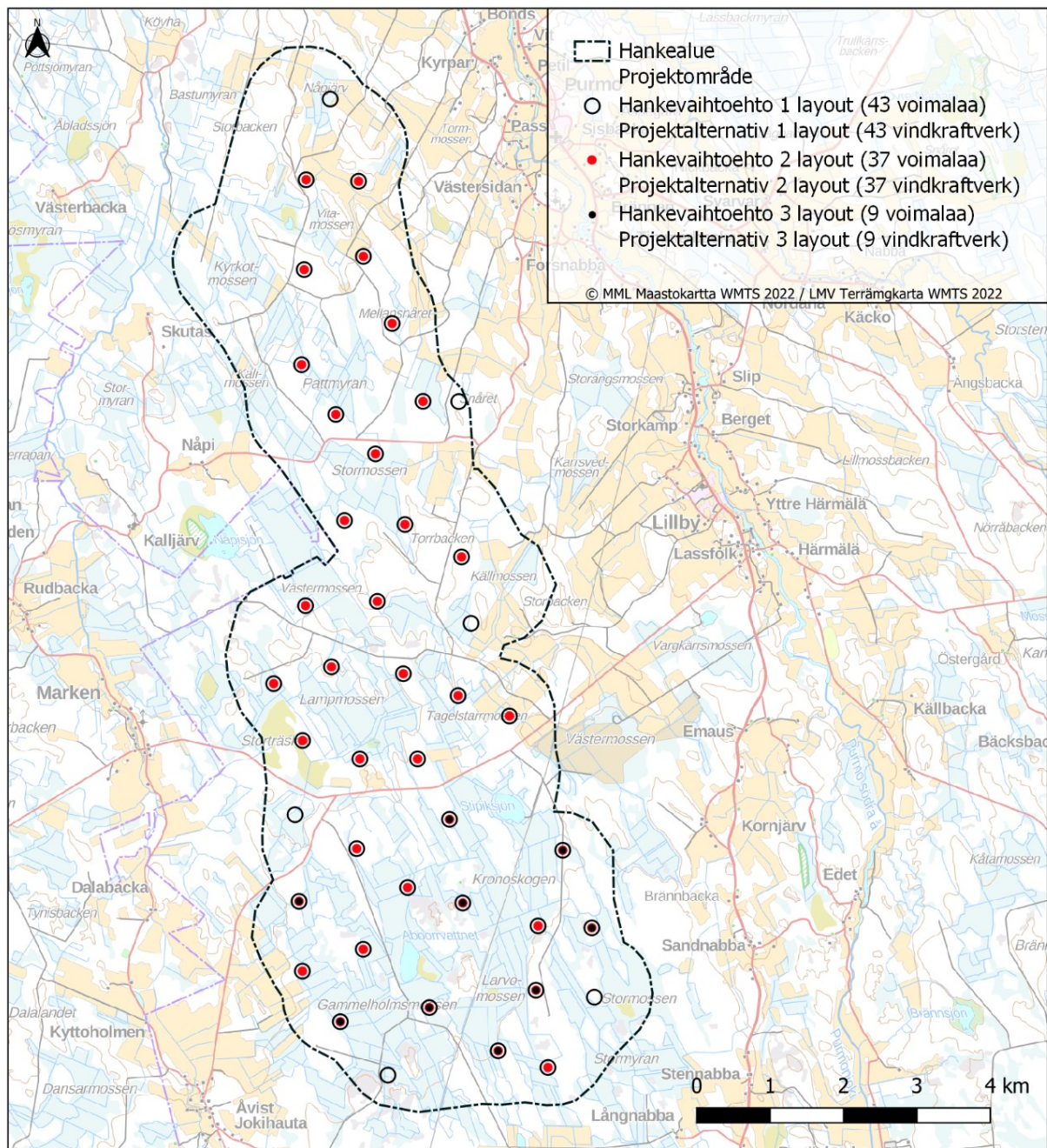
Kuva 1. Purmon tuulivoimapuiston voimalasijoittelu hankevaihtoehdoissa VE1, VE2 ja VE3.
